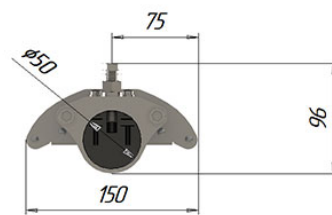
Светильник УСС-50 Катана Трасса ШБ-3; консольное крепление
