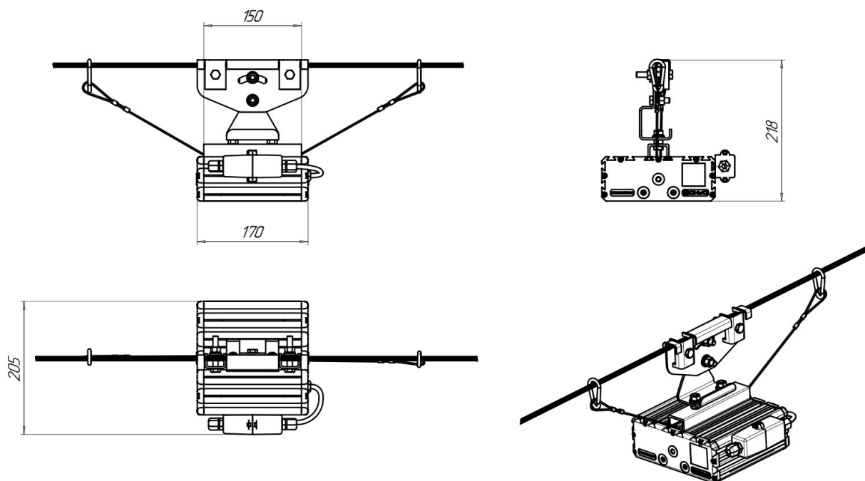
Светильник УСС-32 с креплением на трос
