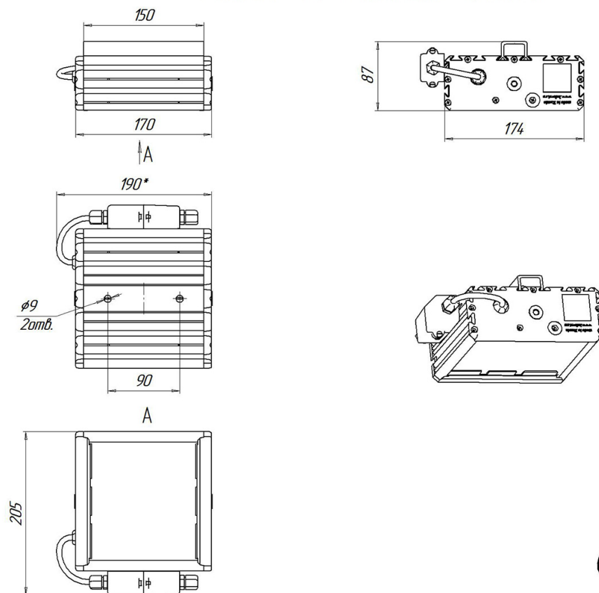
Светильник УСС-32 накладное крепление
