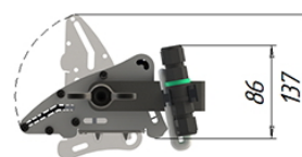
Светильник УСС-200 Эксперт Slim; крепление скоба, IP67
